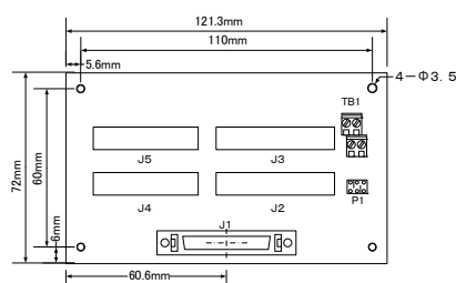
/MS 寸法図
