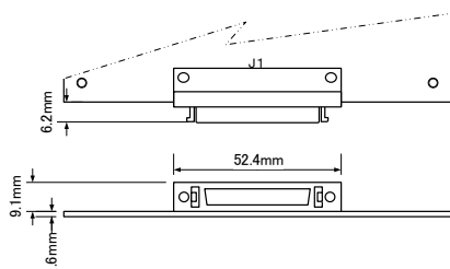
/MR 寸法図
