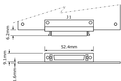
/MR 寸法図
