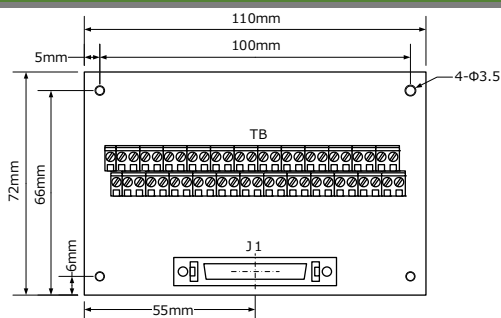
/MS,/MS(D)寸法図
